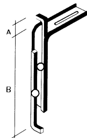
Montážní držák krycího plechu
