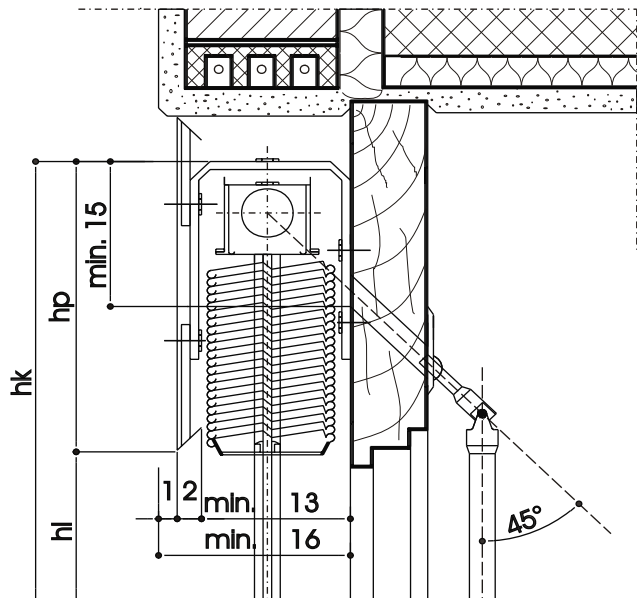
EZ 90 - vertikální řez - montáž s galerií-plechem
