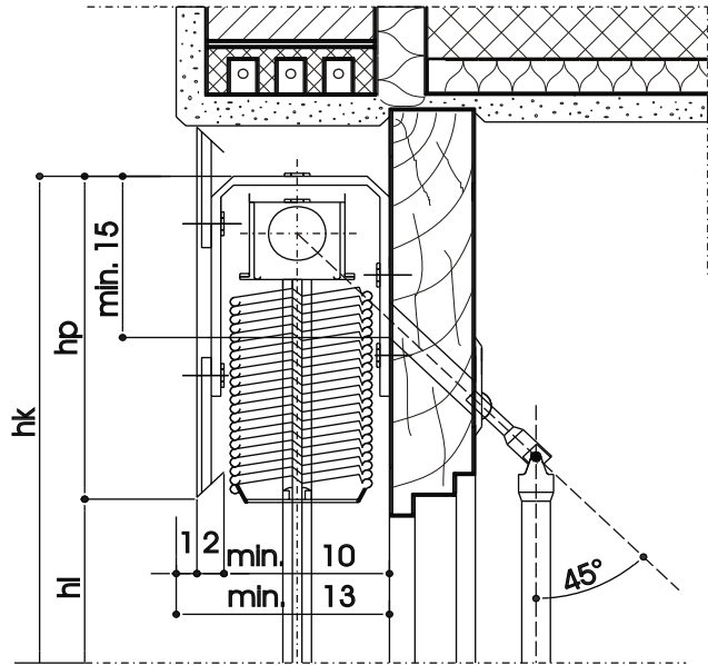
EZ 70 - Vertikalschnitt - Montage mit Deckgalerie
