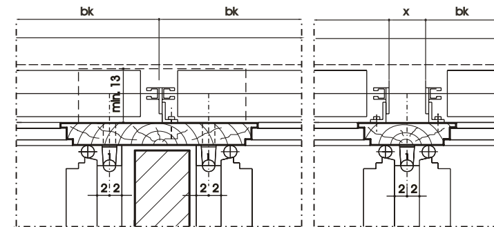
EZ 70 - Horizontalschnitt - Montage auf Fassade
