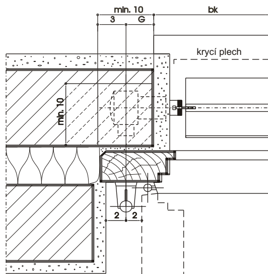
EZ 70 - Horizontalschnitt - Montage in Sturz
