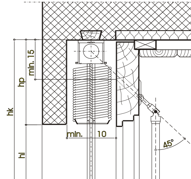
EZ 70 - Vertikalschnitt - Montage in Hohlsturz
