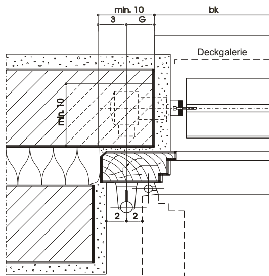
EC 65 - Horizontalschnitt - Montage in Leibung
