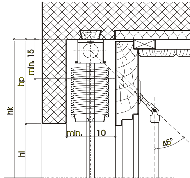
EC 65 - Vertikalschnitt - Montage in Hohlsturz
