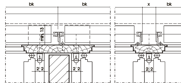
EC 65 - Horizontalschnitt- Montage vor Fassade
