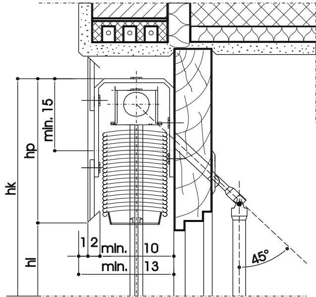
EC 65 - Vertikalschnitt - Montage mit Deckgalerie
