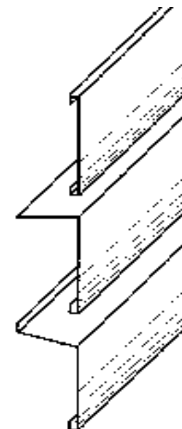
Příkladů tvarů galerií - krycích plechů
